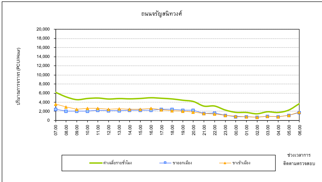
การเปลี่ยนแปลงปริมาณการจราจรตลอดระยะเวลา 24 ชั่วโมง บริเวณถนนเจริญสุนทวงศ์ เดือนมีนาคม 2563
