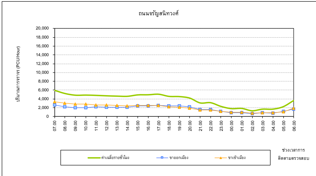
การเปลี่ยนแปลงปริมาณการจราจรตลอดระยะเวลา 24 ชั่วโมง บริเวณถนนเจริญสนิทวงศ์ เดือนกุมภาพันธ์ 2563
