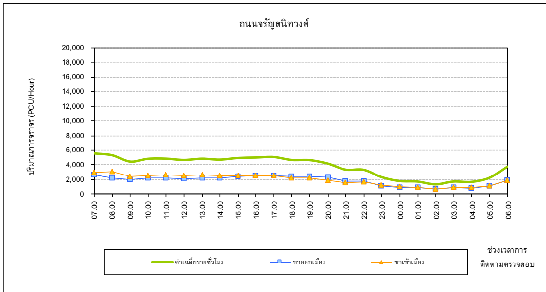
การเปลี่ยนแปลงปริมาณการจราจรตลอดระยะเวลา 24 ชั่วโมง บริเวณถนนจรัญสนิทวงศ์ เดือนมกราคม 2563
