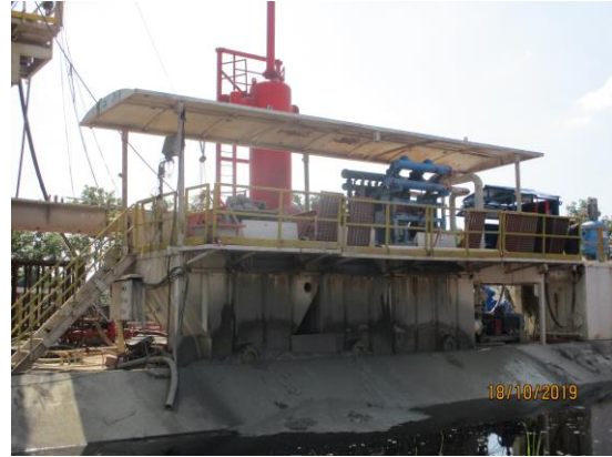
รูปที่ 1-2 ฐานหลุมผลิต L53-B ในระยะเจาะหลุมปิโตรเลียม
