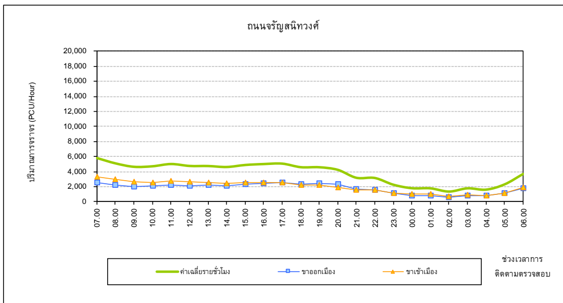
การเปลี่ยนแปลงปริมาณการจราจรตลอดระยะเวลา 24 ชั่วโมง บริเวณถนนเจริญสนิทวงศ์ เดือนตุลาคม 2562
