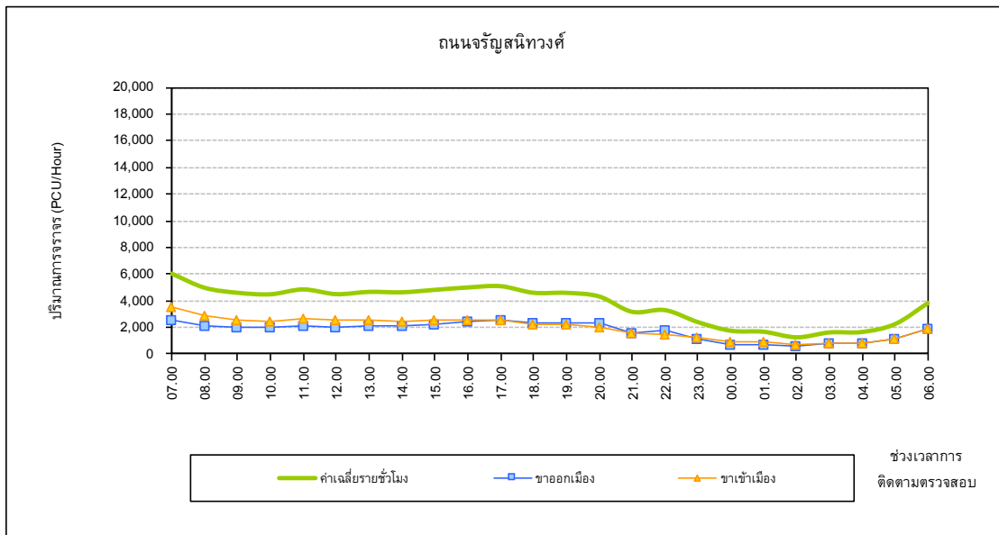
การเปลี่ยนแปลงปริมาณการจราจรตลอดระยะเวลา 24 ชั่วโมง บริเวณถนนเจริญสนิทวงศ์ เดือนกันยายน 2562
