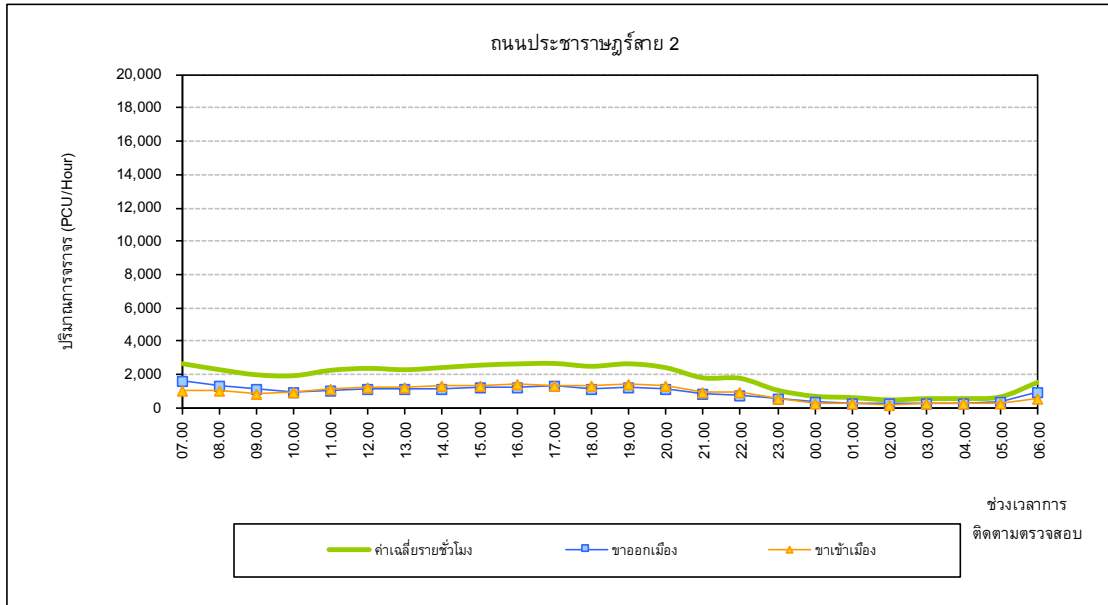
การเปลี่ยนแปลงปริมาณการจราจรตลอดระยะเวลา 24 ชั่วโมง บริเวณถนนประชาราษฎร์สาย 2 เดือนธันวาคม 2562
