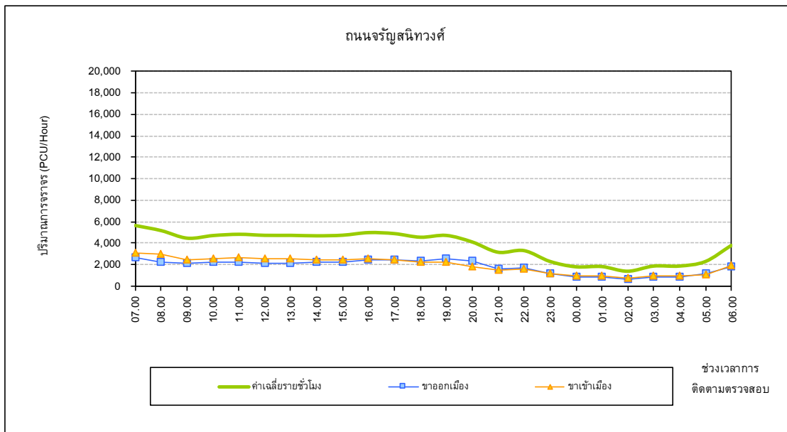
การเปลี่ยนแปลงปริมาณการจราจรตลอดระยะเวลา 24 ชั่วโมง บริเวณถนนจรัญสนิทวงศ์ เดือนธันวาคม 2562
