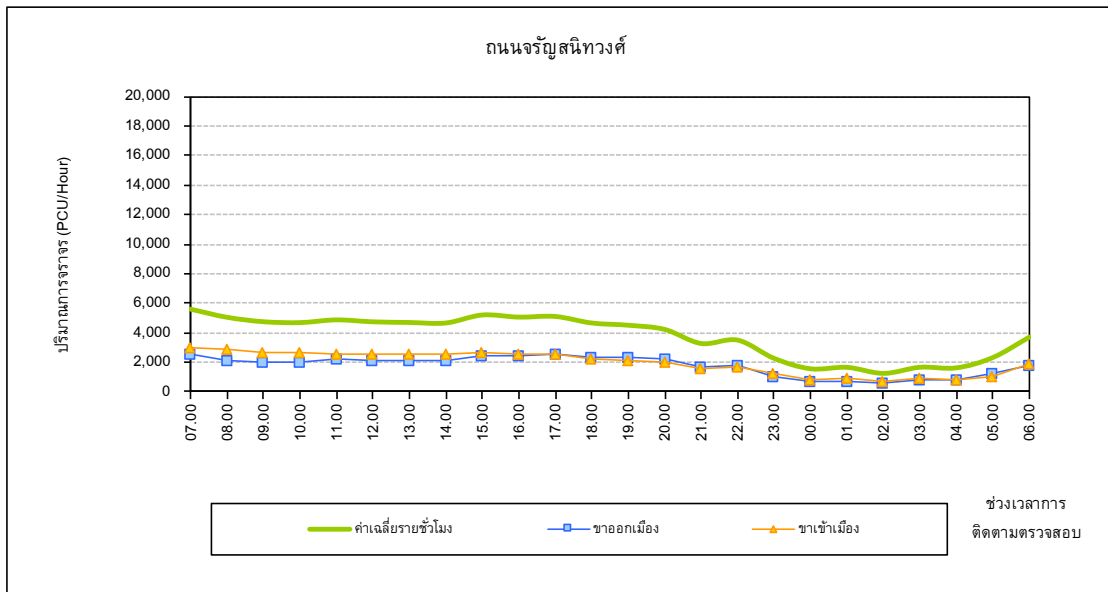
การเปลี่ยนแปลงปริมาณการจราจรตลอดระยะเวลา 24 ชั่วโมง บริเวณถนนเจริญสนิทวงศ์ เดือนกรกฎาคม 2562
