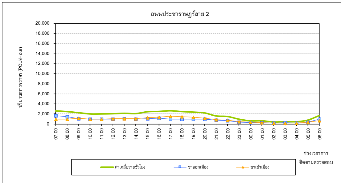
การเปลี่ยนแปลงปริมาณการจราจรตลอดระยะเวลา 24 ชั่วโมง บริเวณถนนพระราชราษฎร์ สาย 2 เดือนตุลาคม 2562
