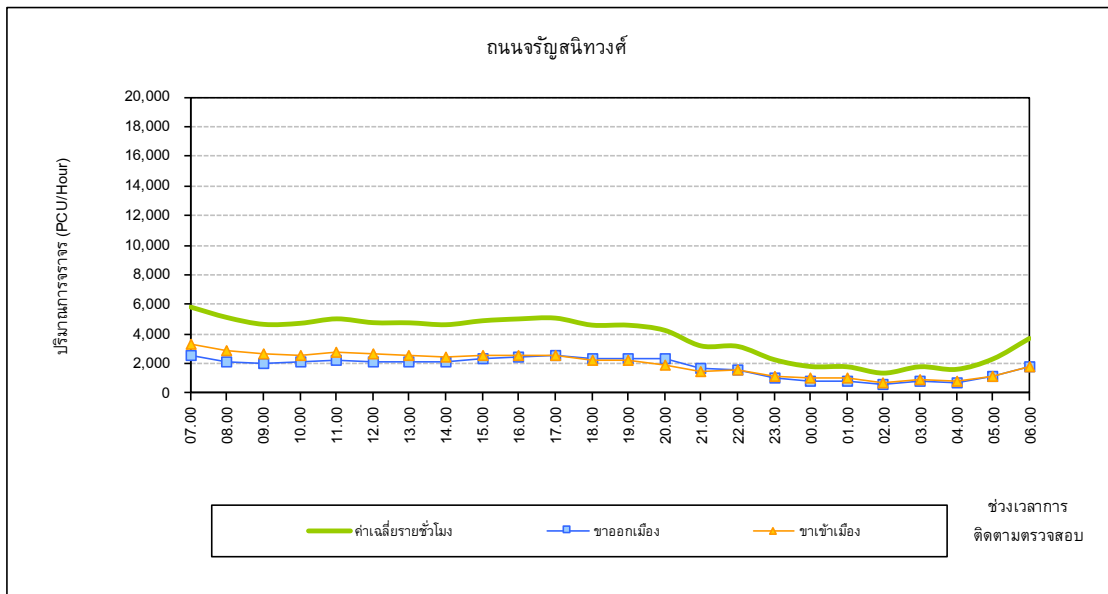
การเปลี่ยนแปลงปริมาณการจราจรตลอดระยะเวลา 24 ชั่วโมง บริเวณถนนจรัญสนิทวงศ์ เดือนพฤศจิกายน 2562
