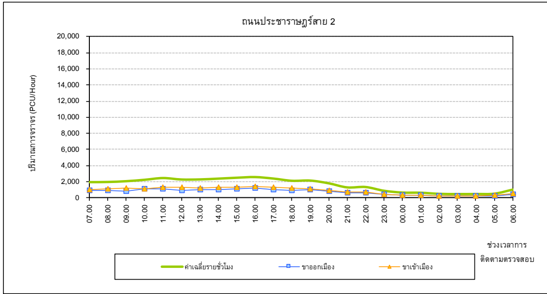
การเปลี่ยนแปลงปริมาณการจราจรตลอดระยะเวลา 24 ชั่วโมง บริเวณถนนพระราชราษฎร์ สาย 2 เดือนกันยายน 2562
